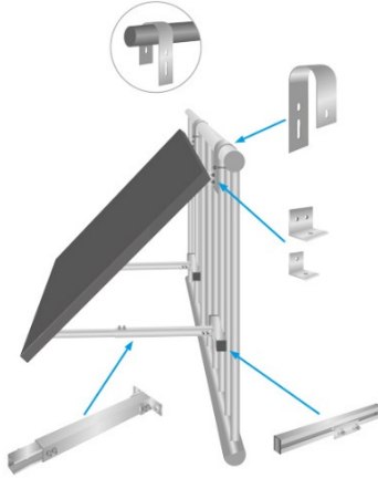
Gitter-Geländer Balkonhalterung
